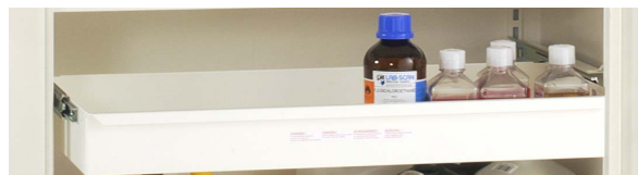
Utdragbar låda, MF4UL Inv. mått: H98 x B850 x D413 mm Kapacitet jämn belastning 80 kg
