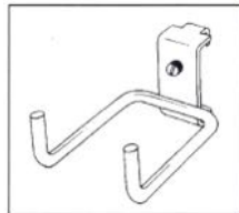
Dubbel Vinkelkrok K3001 Ø 5 x B30 x L 30 mm K3002 Ø 5 x B30 x L 45 mm K3003 Ø 5 x B45 x L 60 mm
